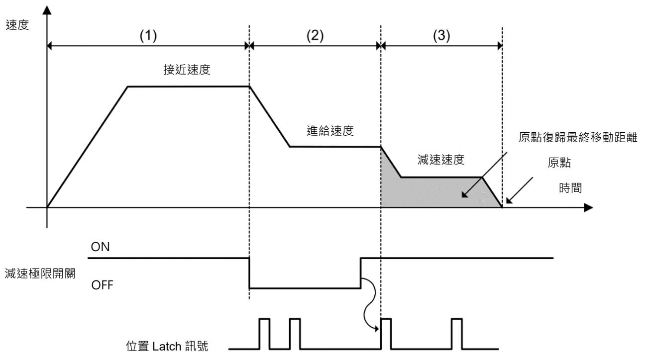
圖 3.2.12.2 原點復歸動作順序 (MODE = 1)
