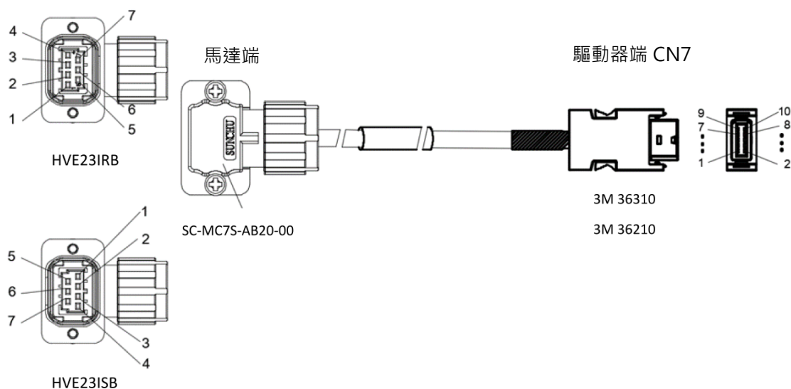
圖16.1.2.5 HVE23IRB□□MB / HVE23ISB□□MB 編碼器延長線（串列增量式，不含電池）
