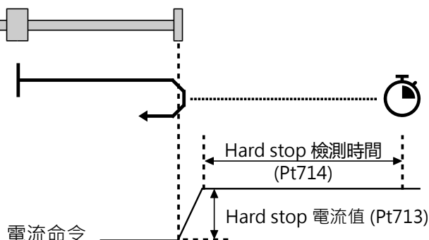
圖8.11.1.4 Hard stop示意圖
