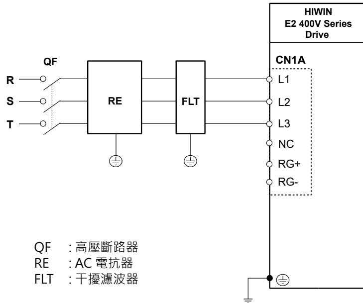
圖5.3.2.6.1 400 V驅動器AC電抗器配線
