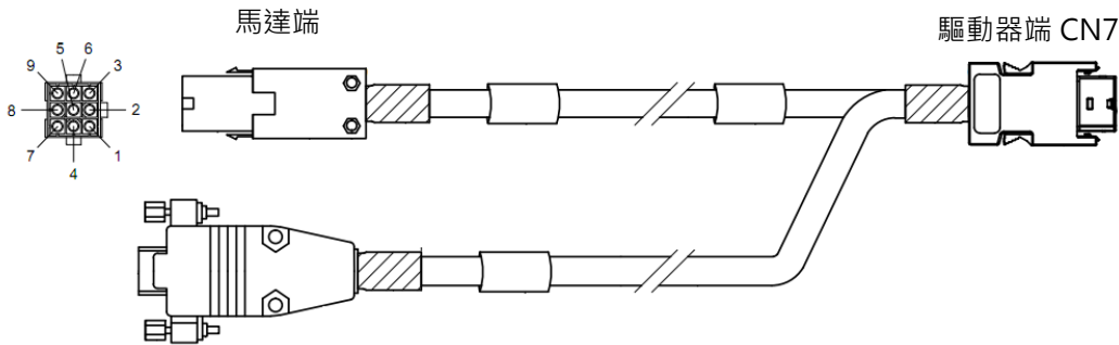
Renishaw BiSS-C 編碼器 ( D-sub 9 PIN )
