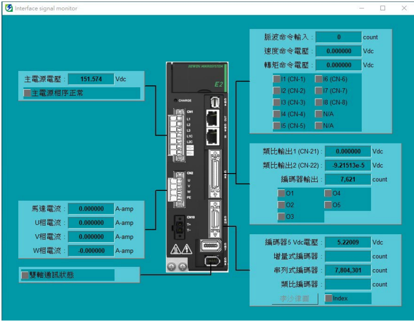
圖11.2.1.1 Interface signal monitor視窗的顯示資訊
