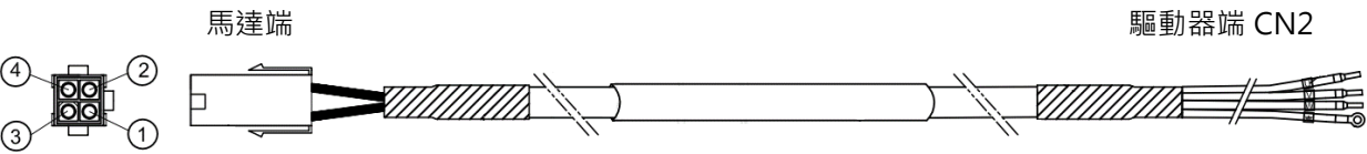
圖16.1.1.1 HVPS04AA□□MB 伺服馬達動力線（不含制動器訊號）
