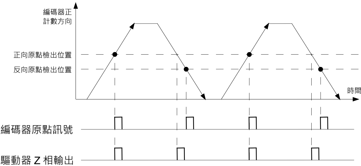
圖 8.6.2.3 Pt70A = t.□□□0，關閉多原點輸出功能
