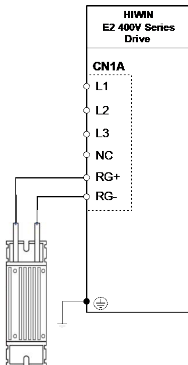
圖5.3.2.5.1 400 V驅動器外部回生電阻配線
