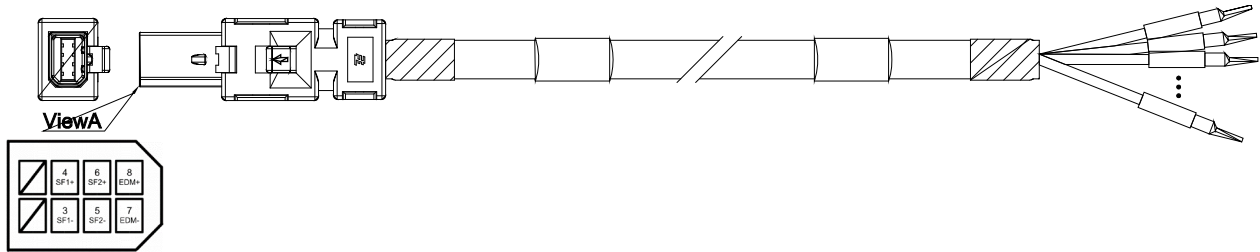
圖 16.1.8.1 STO 訊號傳輸線
