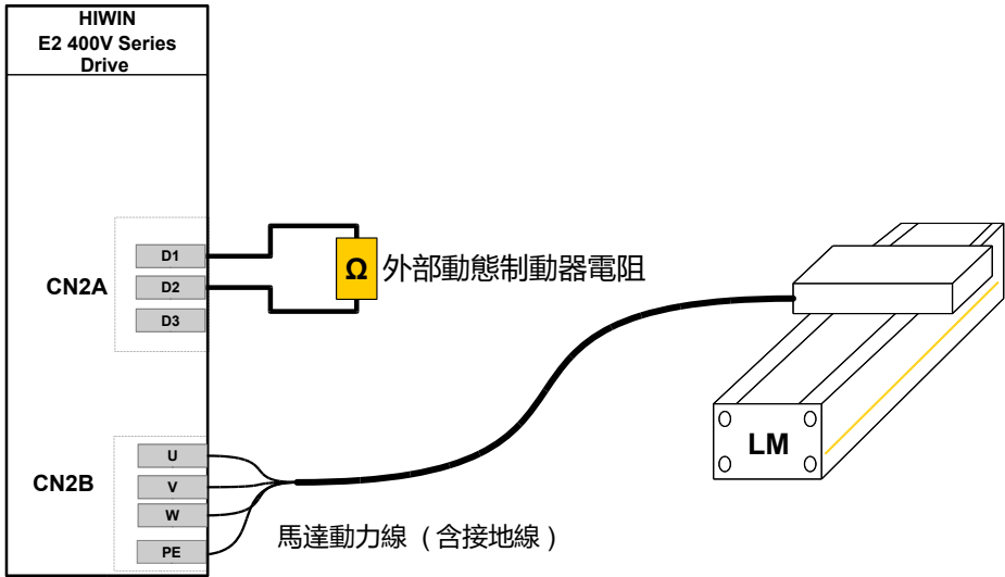
圖5.4.4.2.4 使用內建動態制動器電路與外部動態制動器電阻
