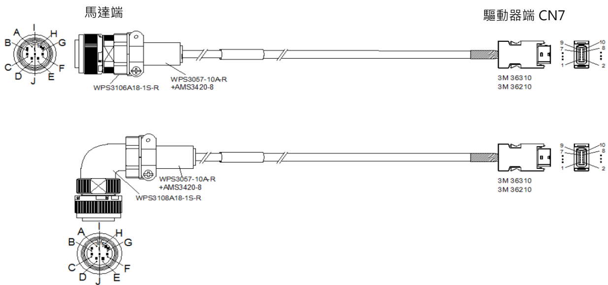
圖16.1.2.3 HVE23IBB□□MB / HVE23ICB□□MB 編碼器延長線 (串列增量式·不含電池)
