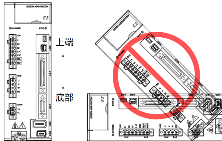
圖4.1.2.1 驅動器擺放示意圖
