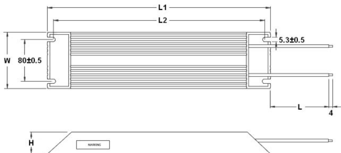
圖16.2.5.2 回生電阻050100700031尺寸圖
