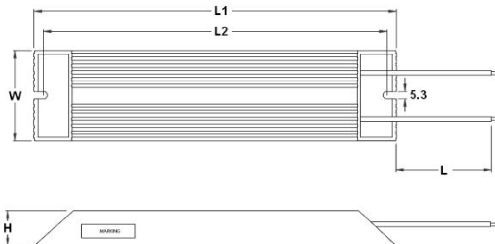
圖16.2.5.1 回生電阻050100700001尺寸圖
