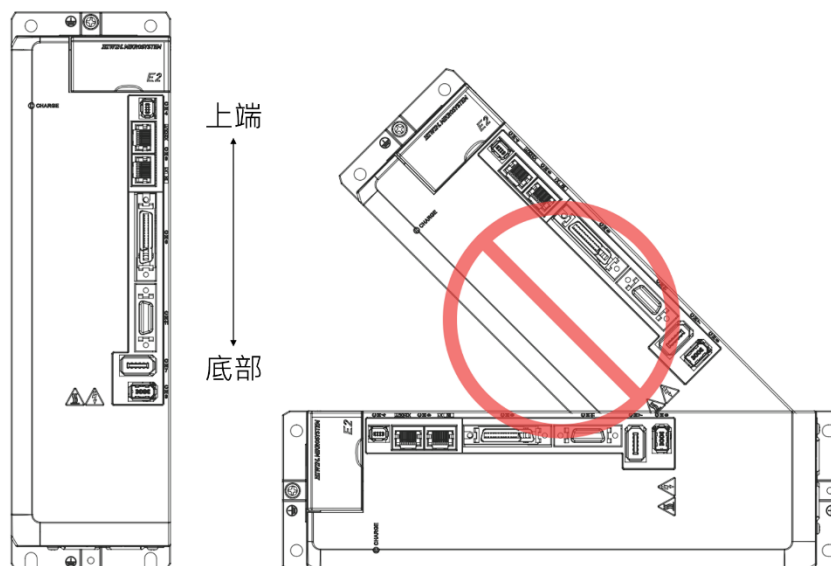
圖4.2.2.1 驅動器擺放示意圖
