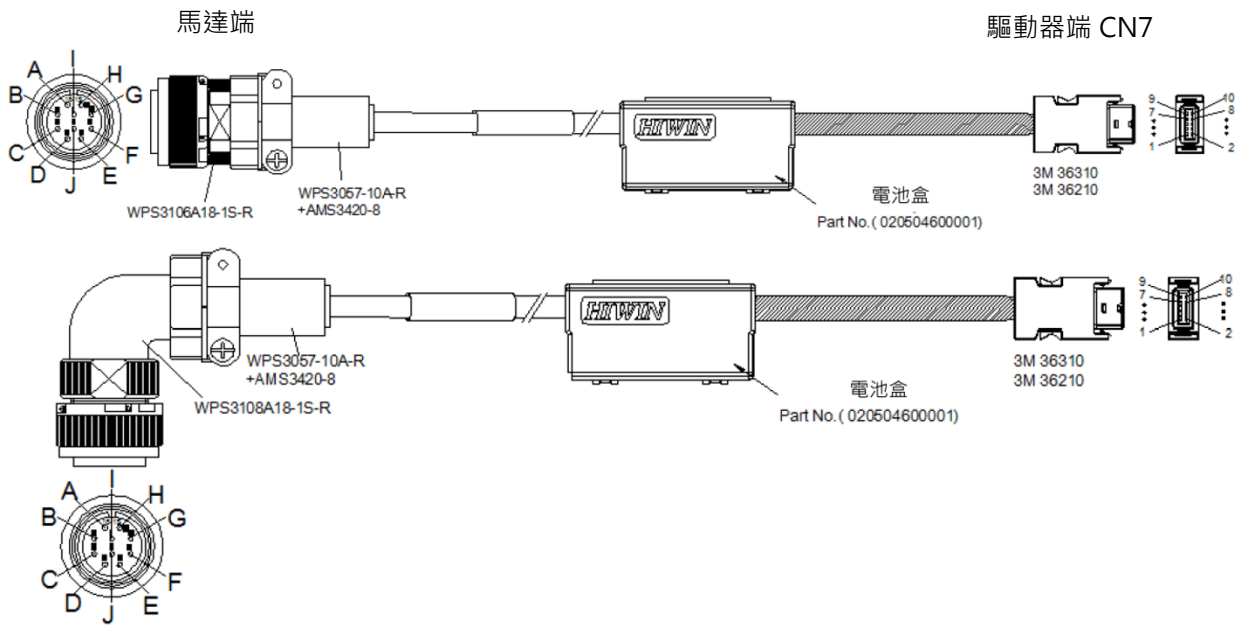
圖16.1.2.4 HVE23ABB□□MB / HVE23ACB□□MB 編碼器延長線 (串列絕對式，含電池)
