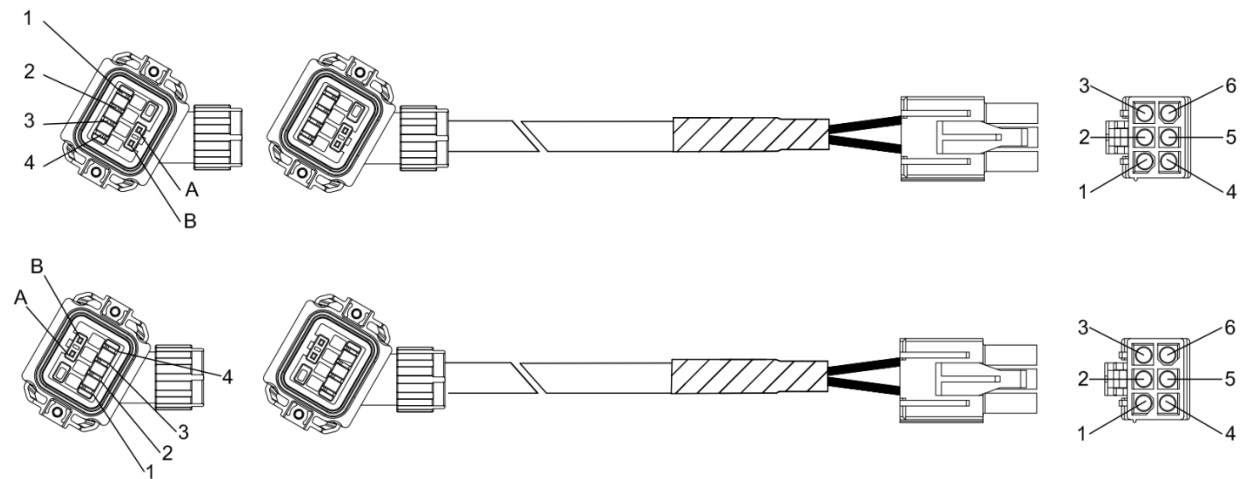
圖16.1.1.6 120600100054 / 120600100055 動力線轉接線材 ( 含制動器訊號 )
