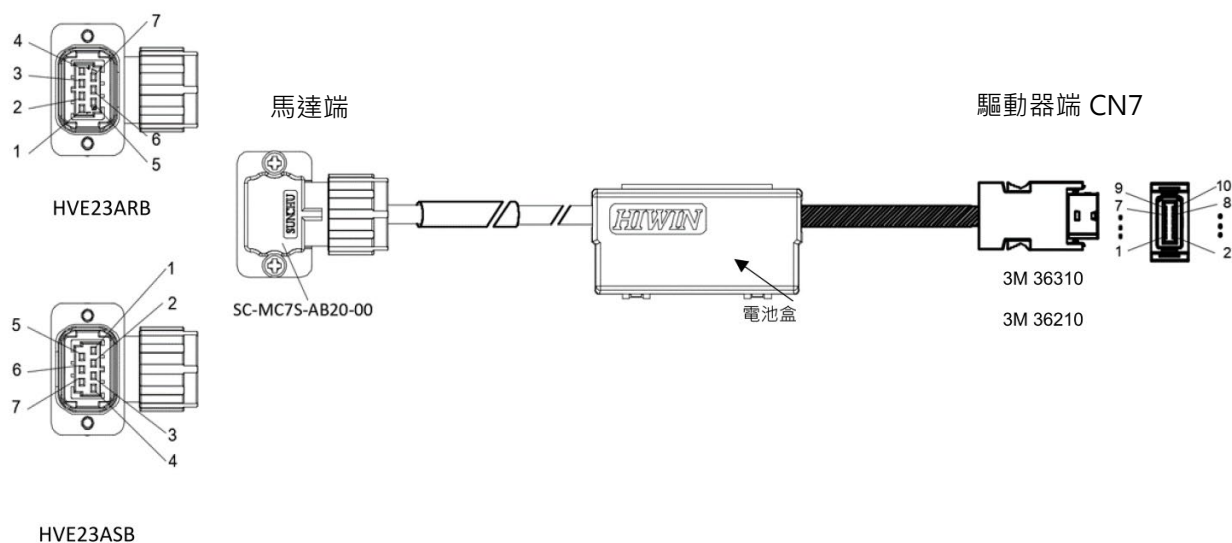
圖16.1.2.6 HVE23ARB□□MB / HVE23ASB□□MB 編碼器延長線（串列絕對式，含電池）
