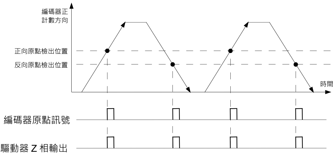
圖 8.6.2.4 Pt70A = t.□□□1，開啟多原點輸出功能
