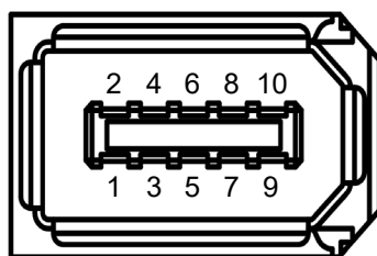
圖5.4.3.1 驅動器端編碼器連接埠示意圖
