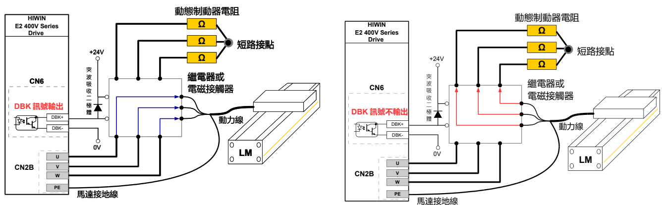
圖5.4.4.2.5 使用外部動態制動器電路與外部動態制動器電阻
