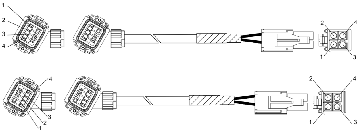
圖16.1.1.5 120600100052 / 120600100053 動力線轉接線材 ( 不含制動器訊號 )
