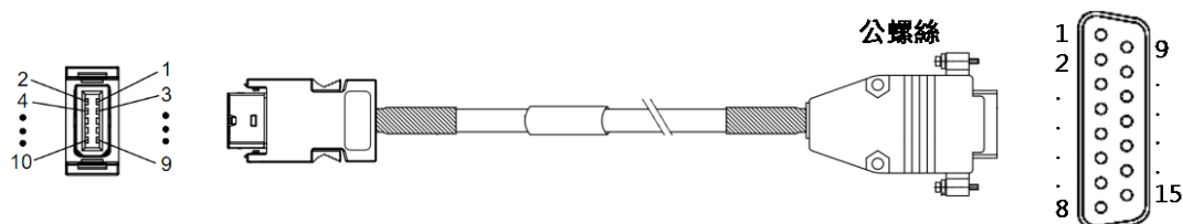
圖 16.1.3.2 HE00817EK□00 編碼器延長線 (Renishaw 數位編碼器用)
