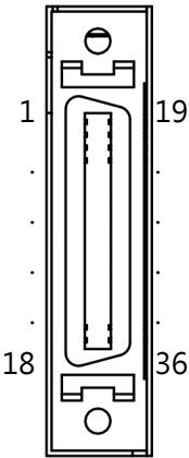
圖5.5.1.2 驅動器端CN6腳位示意圖-總線型 (ED2F)
