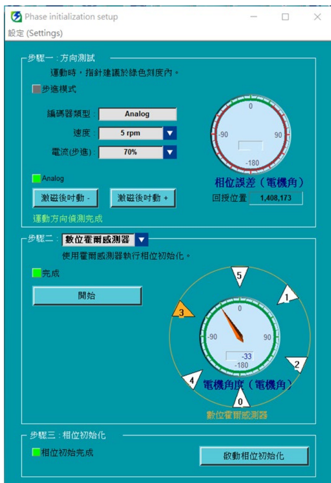
圖7.5.3.1 數位霍爾感測器操作流程
