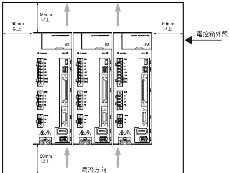
圖4.1.2.2 多台驅動器的安裝示意圖
