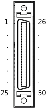
圖5.5.1.1 驅動器端CN6腳位示意圖-標準型 (ED2S)
