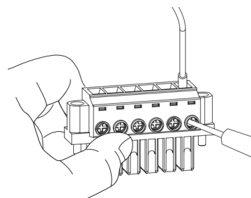
十字螺絲刀的使用方法
