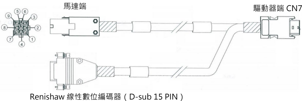
圖16.1.2.7 HE00817DR□00 編碼器延長線 (串列增量式，全閉環控制適用，不含電池)
