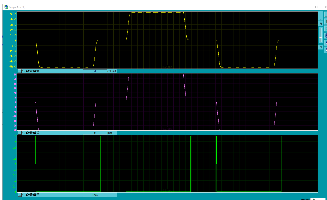
圖 11.3.2.1 由 Scope 觀察運動狀態
