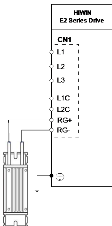
圖5.3.1.5.1 110 V / 220 V驅動器外部回生電阻配線
