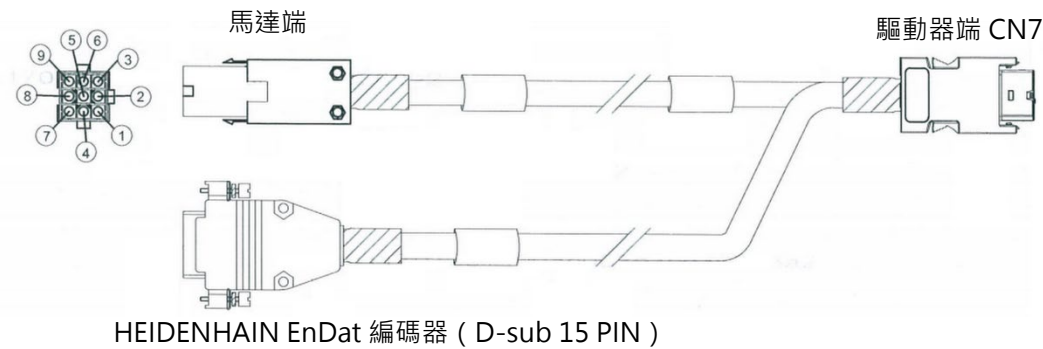
圖16.1.2.10 HE00EKDDJ□00 編碼器延長線（全閉環控制適用，不含電池）
