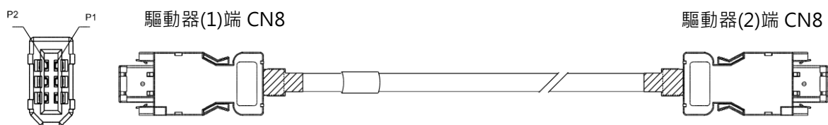
圖16.1.7.2 驅動器龍門通訊線
