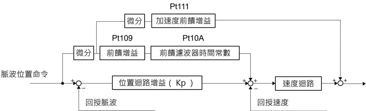
圖10.7.1.1 前饋命令控制架構
