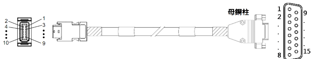
圖16.1.3.1 HE00EJ6DF□00 編碼器延長線 (Renishaw數位編碼器用)
