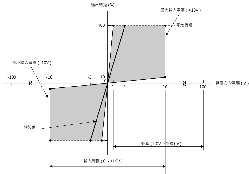
圖8.5.1.2 轉矩命令電壓輸入範圍
