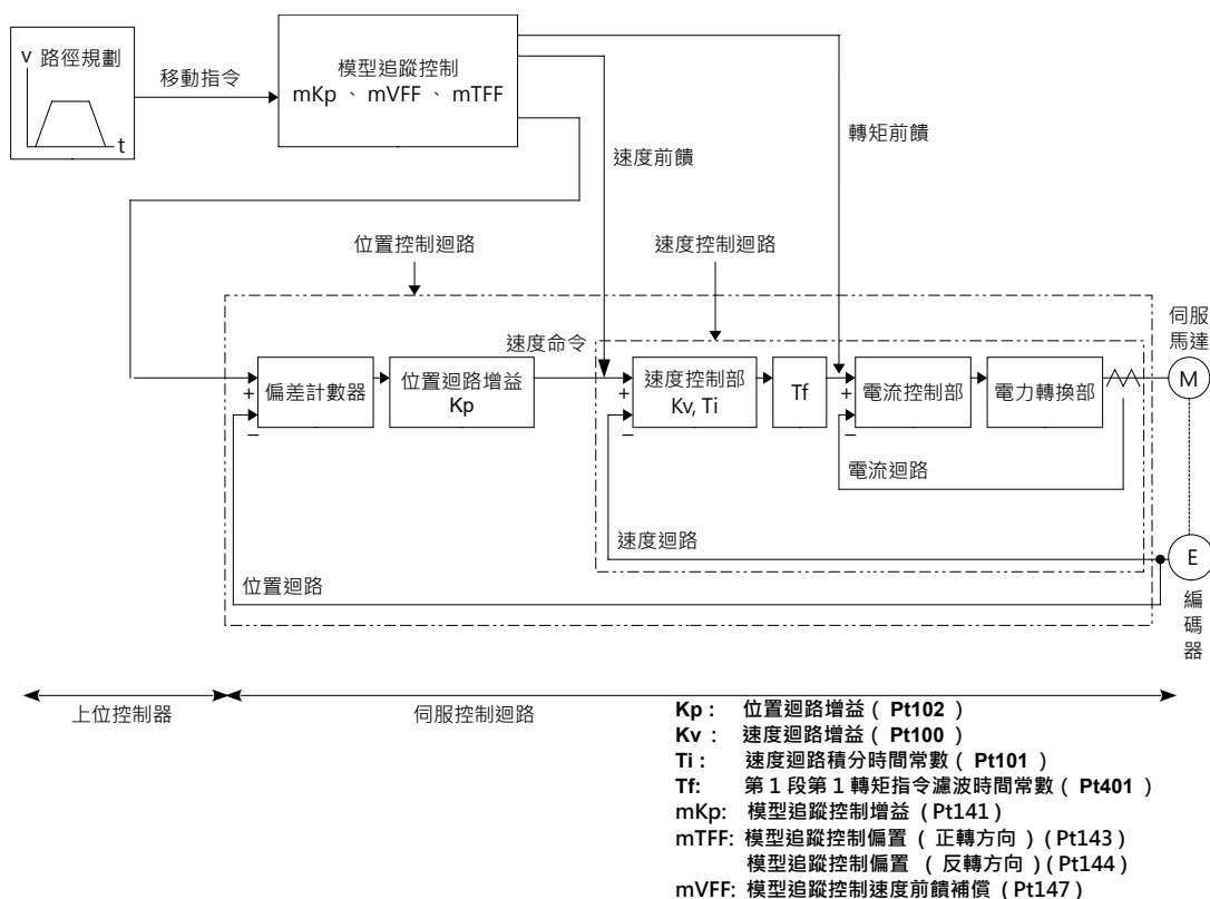
圖10.6.8.1 追蹤控制方塊圖
