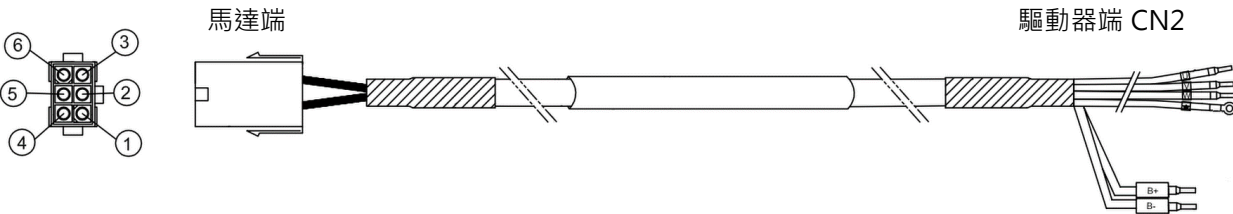
圖16.1.1.2 HVPS06AA□□MB 伺服馬達動力線（含制動器訊號）
