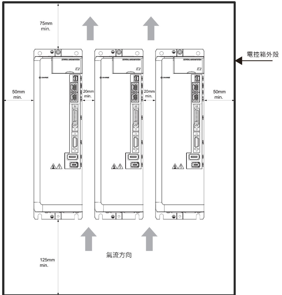
圖4.2.2.2 多台驅動器的安裝示意圖
